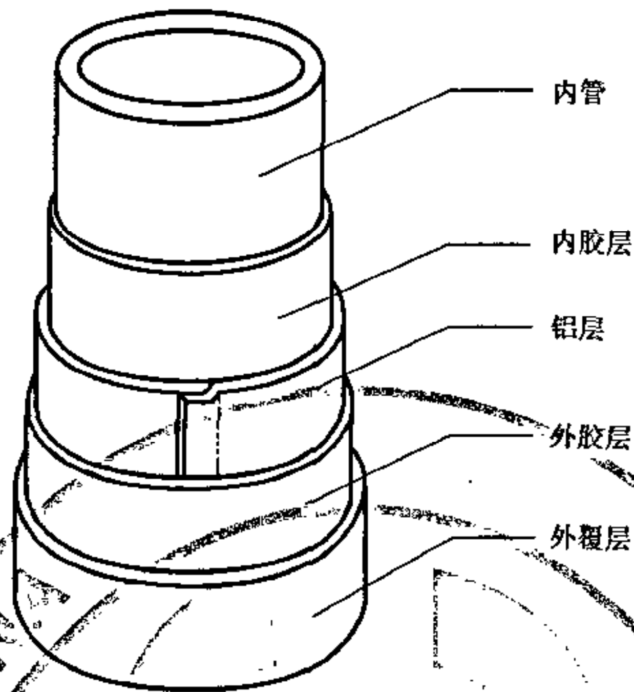
图 1 无规共聚聚丙烯(PP-R)塑铝稳态复合管五层结构示意图
