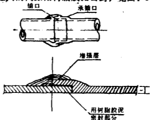
图 4-3-2 承插式连接
