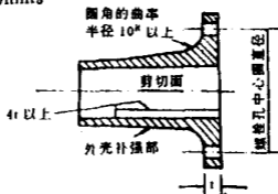
图 4-3-3 法兰剖面
