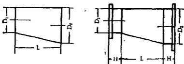
偏心异径管
